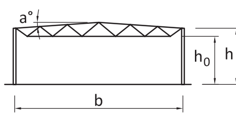
Post-ferm konstruktsiooniga standardhall
